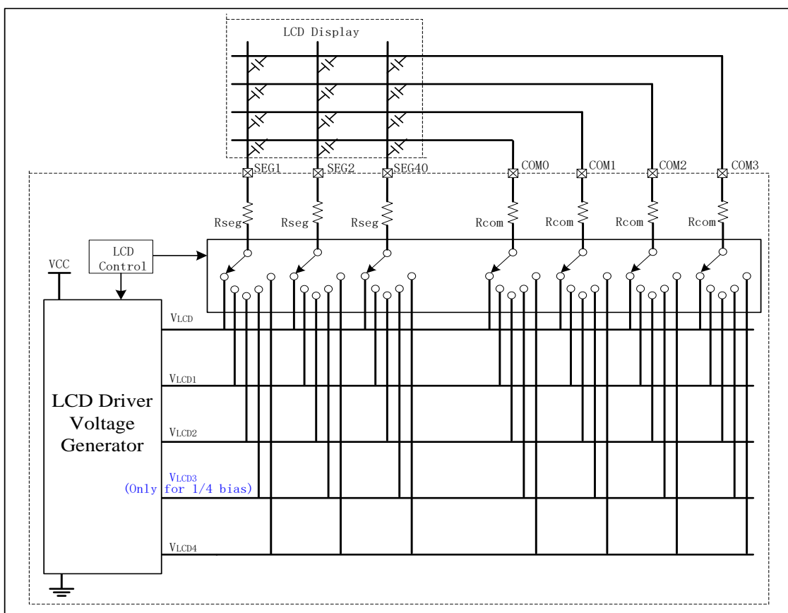
LCD 模块功能框图
