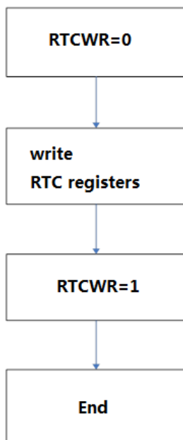
RTC 指示寄存器写流程
